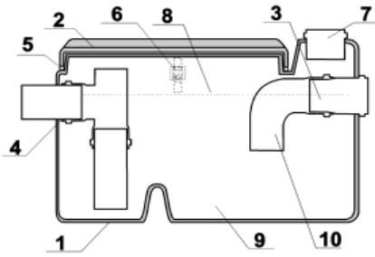
Принципиальная схема жиросепаратора серии СЖ "Оптима"
